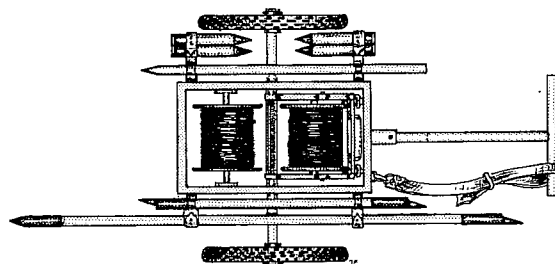
Fernsprechkarren mit verlastetem Baumaterial
