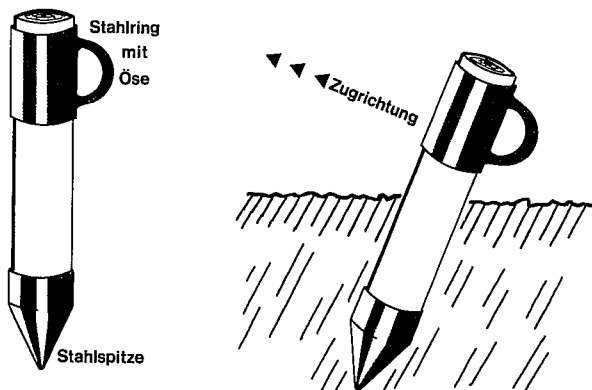
Ankerpfahl/Ankerseil
