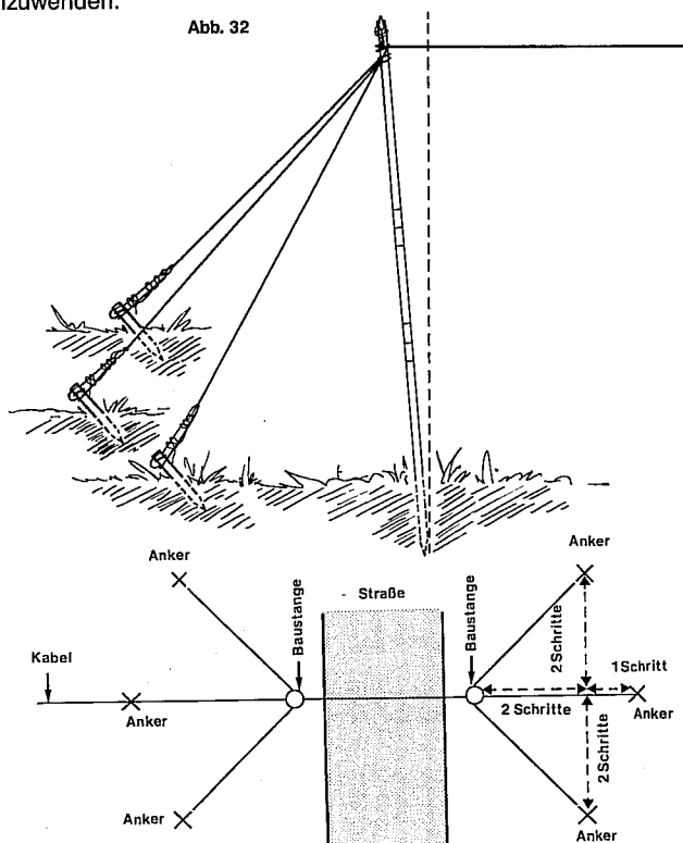
Dreifach-Anker
