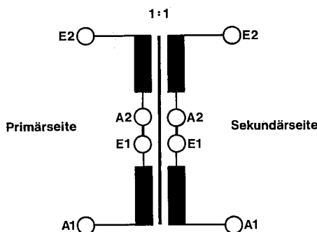
Schaltbild
