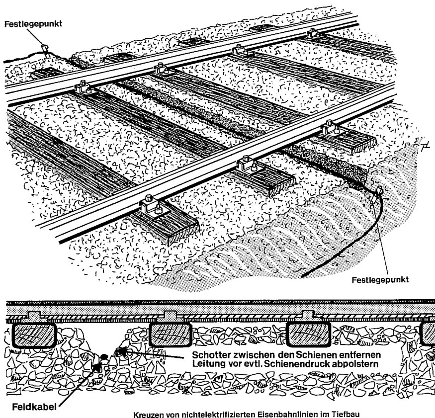
Kreuzen von nichtelektrifizierten Eisenbahnlinien im Tiefbau
