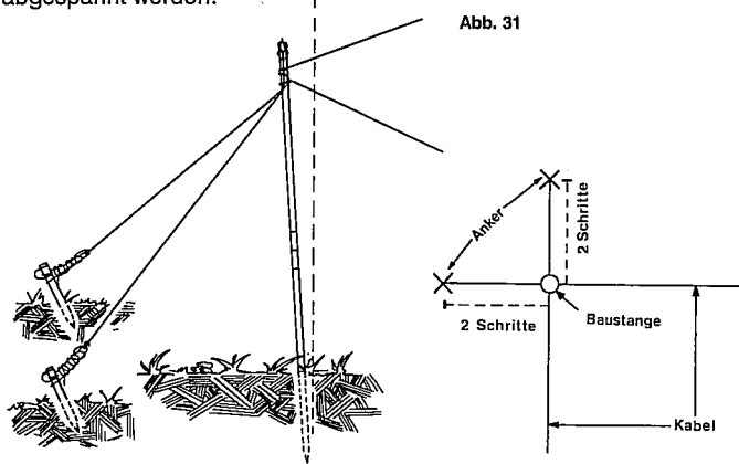
Zweifach-Anker
