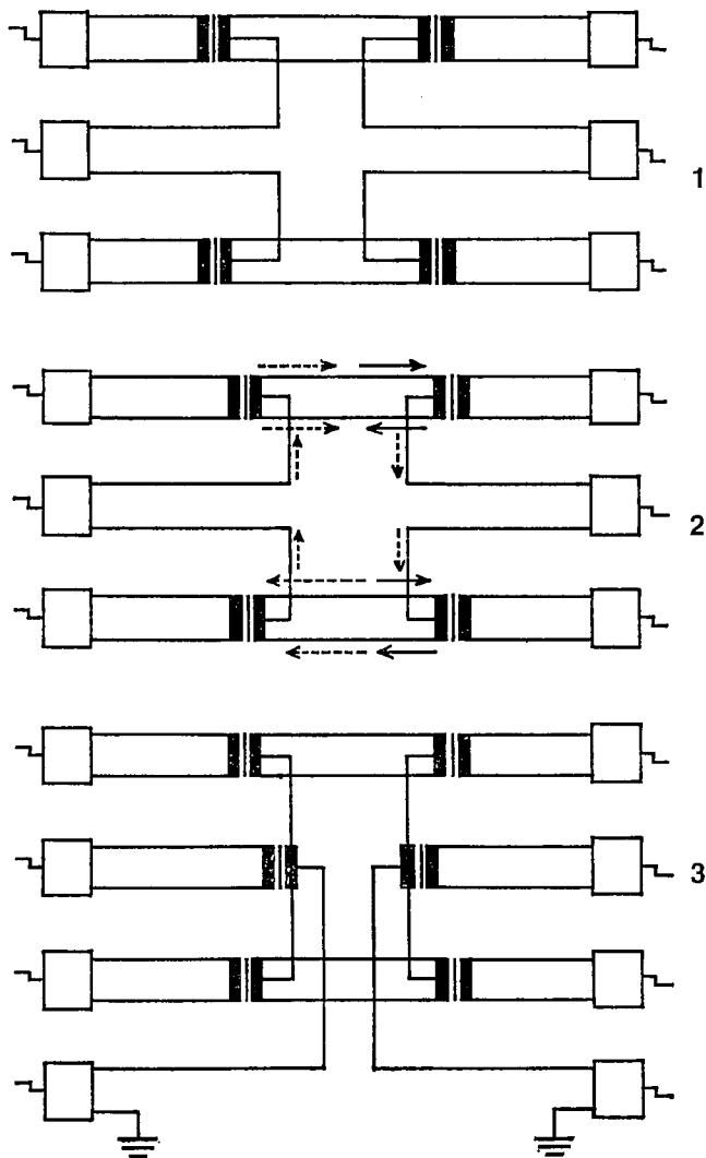
Ringübertrager — Schaltungen
