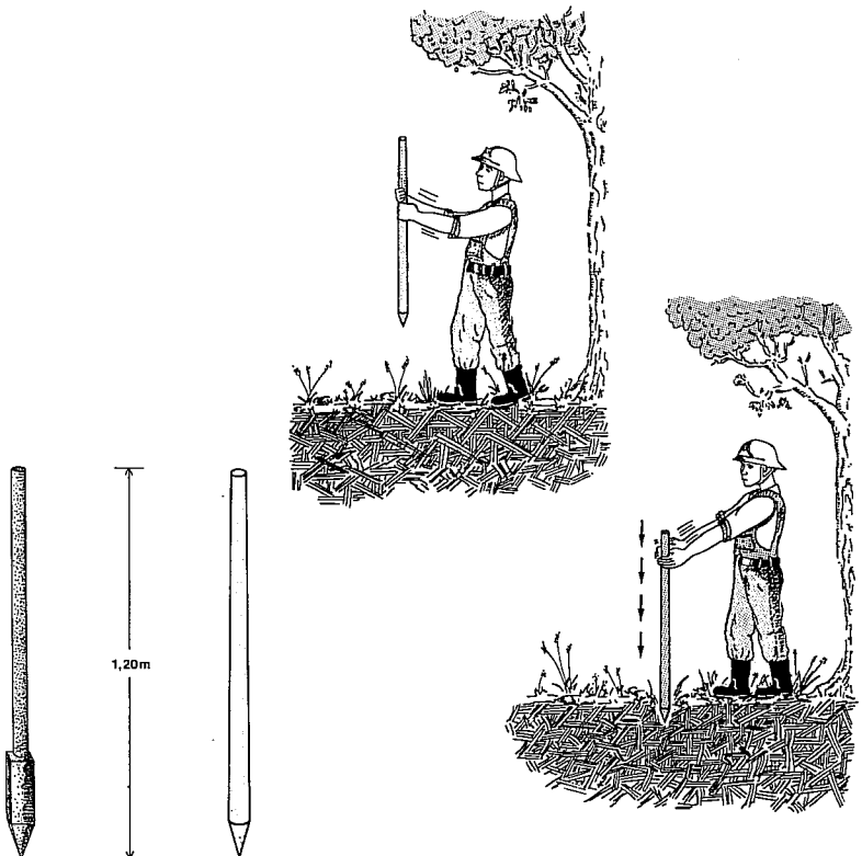
Pfahleisen/Handhabung des Pfahleisens
