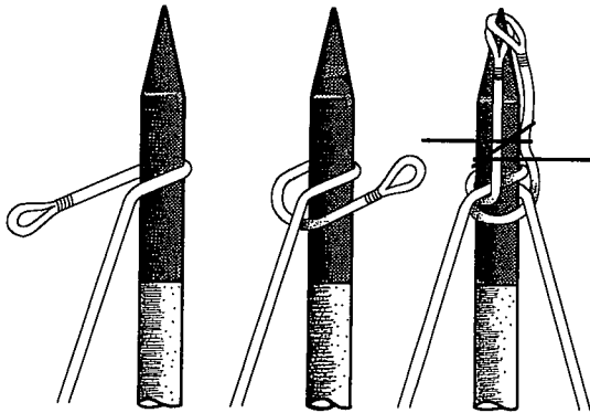
Befestigen des Ankerseils an der Baustangenspitze
