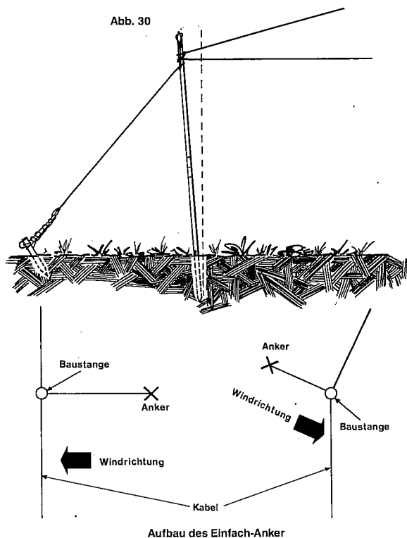
Aufbau des Einfach-Anker
