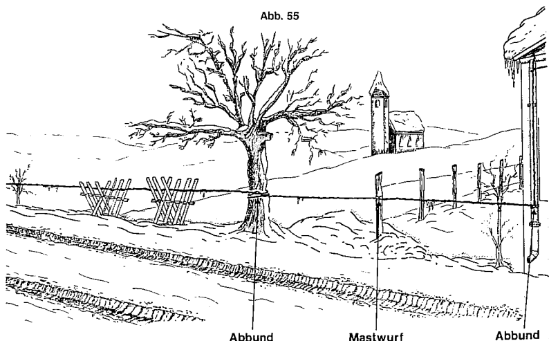
Verlegen des Feldkabels bei Schnee
