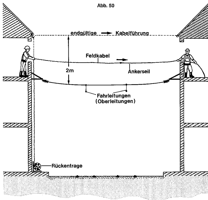
Kreuzen von Fahrleitungen (Oberleitungen)
