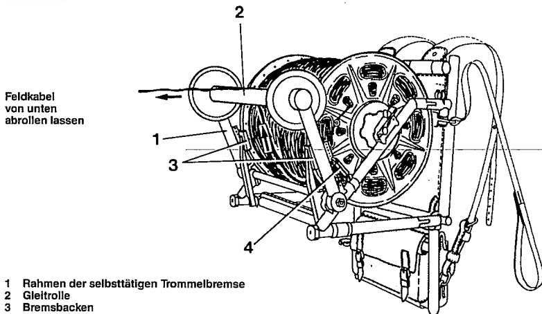
Auslegen mit Trommelbremse, selbsttätig
