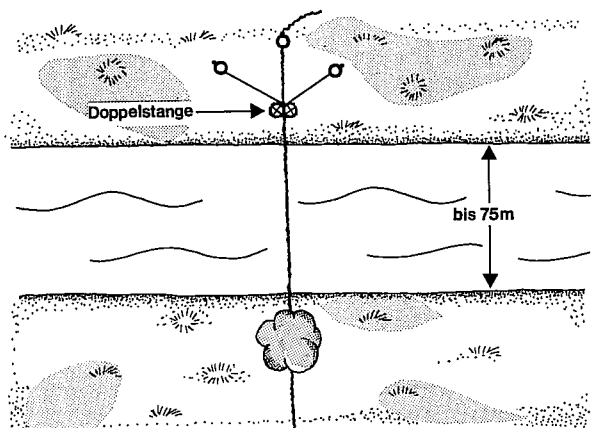
Überspannen von Gewässern
