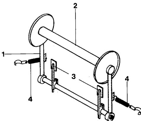
Trommelbremse, selbsttätig
