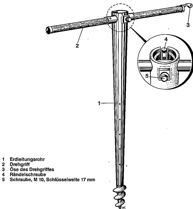
Erdleitungsrohr
