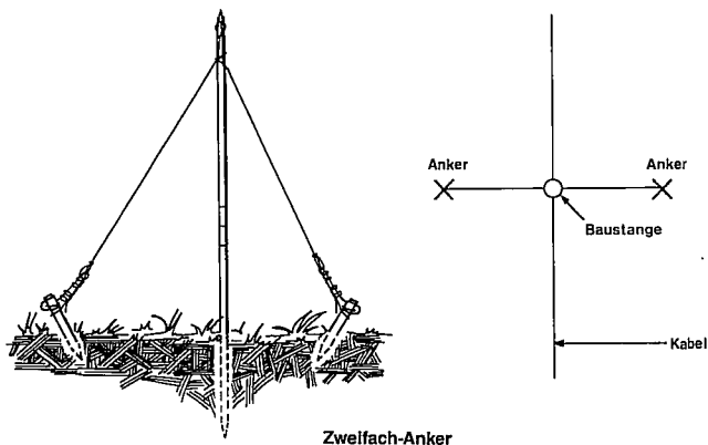
Zweifach-Anker
