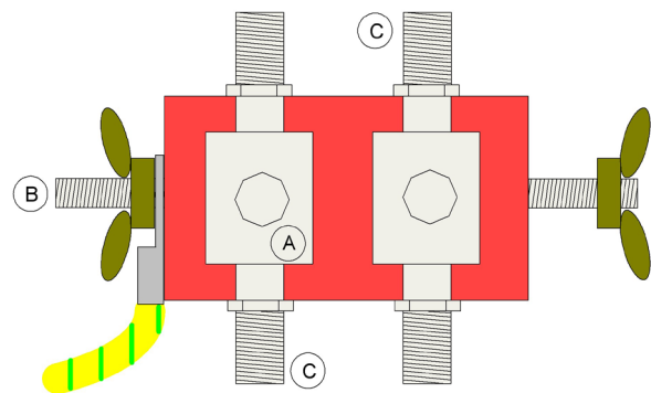
Bild 7: Metallene HF-Kabelbox
